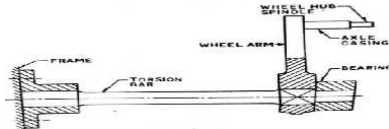
Torsion bar
